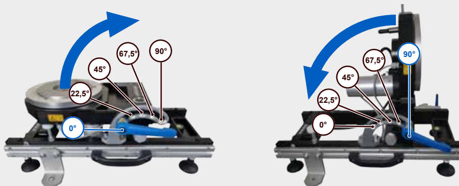
Schwenkplatte in 5 Positionen einstellbar (0-90°).
